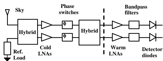
Figura 1. Diagrama de bloques del radiómetro Planck.
